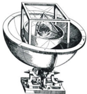
Keplers Modell der relativen Größen der Planetenbahnen (Mysterium Cosmographicum, 1596)
